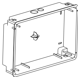
touchDock mini: Boite d'encastrement avec cadre Aluminum (1)
