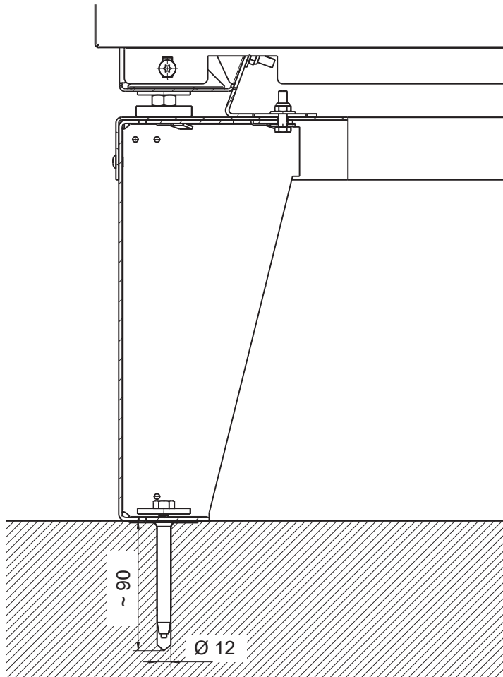
Mit Unterbau (UO/UG) / Wiegesockel (WI)
