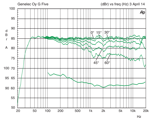
Abbildung 6. Die obere Kurvenschar zeigt die horizontale Abstrahlcharakteristik des G Five gemessen in einem Meter Abstand. Die untere Kurve zeigt das Bündelungsmaß.
