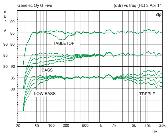
Bild 7. "Kurvorna visar effekten av "Tabletop", "Bass", "Low Bass" och "Treble"-inställningarna på frekvenskurvan hos G Five i fritt rum.
