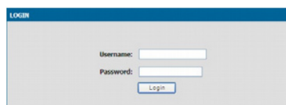
Рис. 6. Сообщение аутентификации
