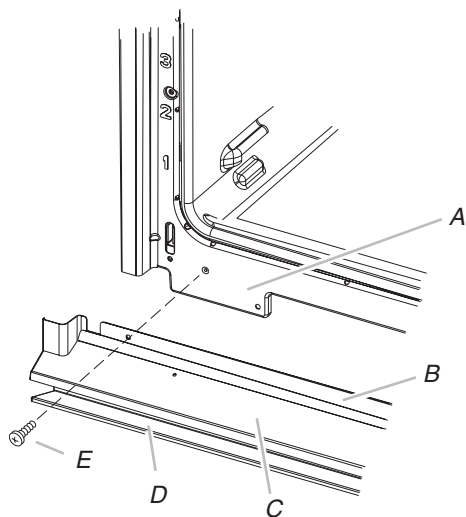
A. Marco del horno B. Lengüeta de ducto de ventilación C. Ducto de ventilación del horno D. Deflector para cajón de calentamiento E. Tornillo n.º 8-18 x 3/8" (9,5 mm)
