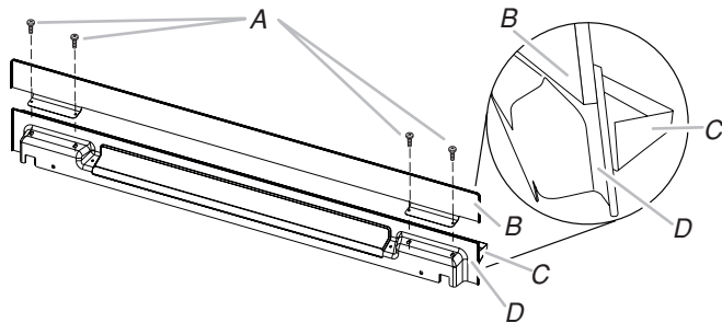
A. Tornillos n.º 8-18 x 1/4" (6,4 mm) B. Deflector para cajón de calentamiento C. Ducto de ventilación
