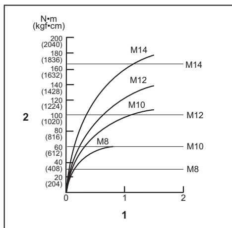
1. Timp de strângere (secunde) 2. Cuplu de strângere
