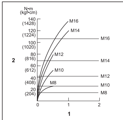
1. Timp de strângere (secunde) 2. Cuplu de strângere
