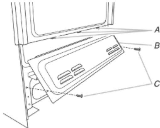
A. Onglets de montage (3) B. Couvercle d'accès inférieur C. Vis (2)
