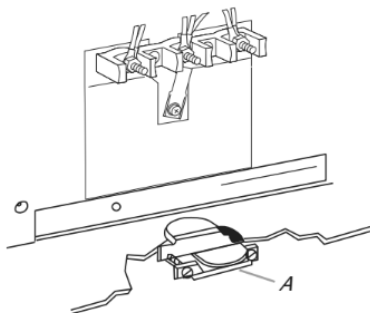
A. Serre-câble (homologation UL)
