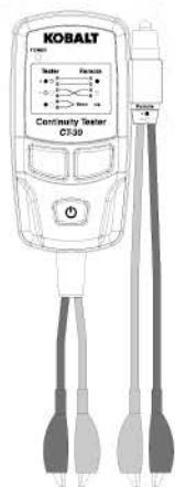
ARTÍCULO #2545075 Probador de continuidad con control remoto MODELO #CT-30
