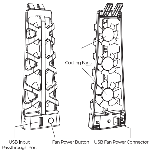
Cooling Fan
