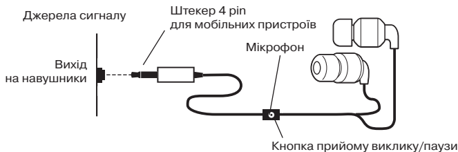
Мал. 1. Схема підключення
