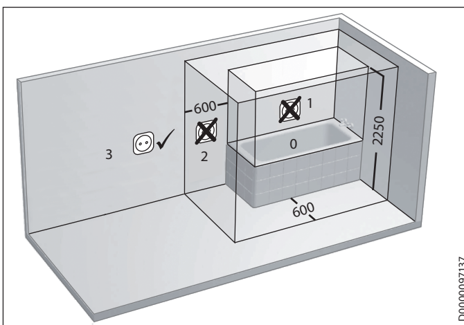
Зоны электрозащиты в ванной комнате
