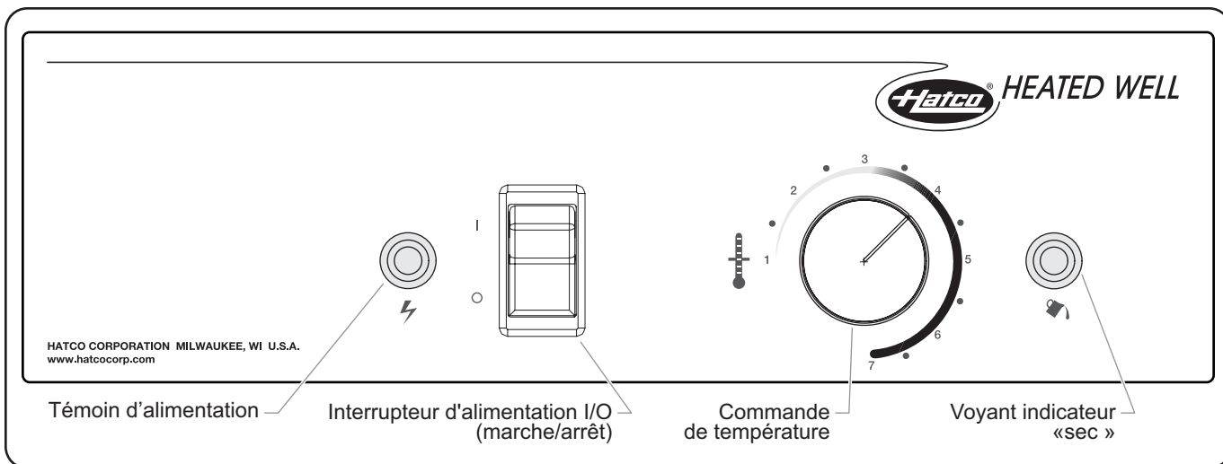
Panneau de contrôle des modèles HW et CHW
