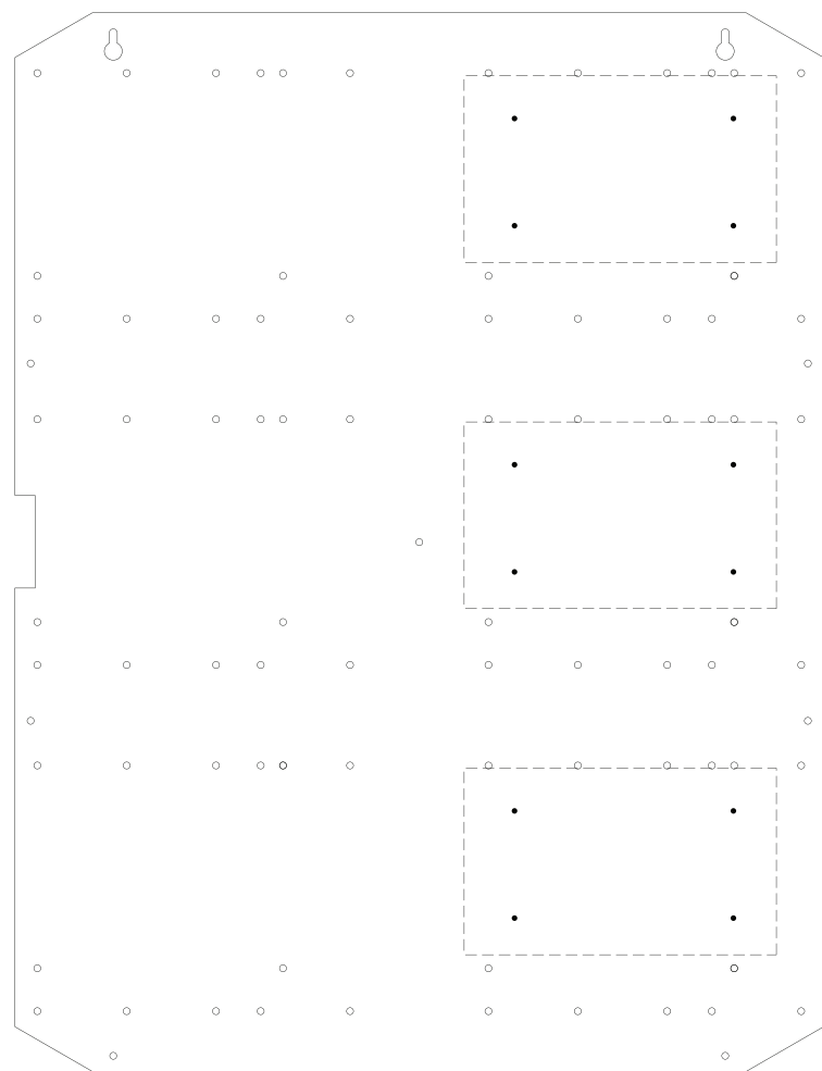
Fig. 4 - TMV2 Mercury/HID/Vertx Door Backplane
