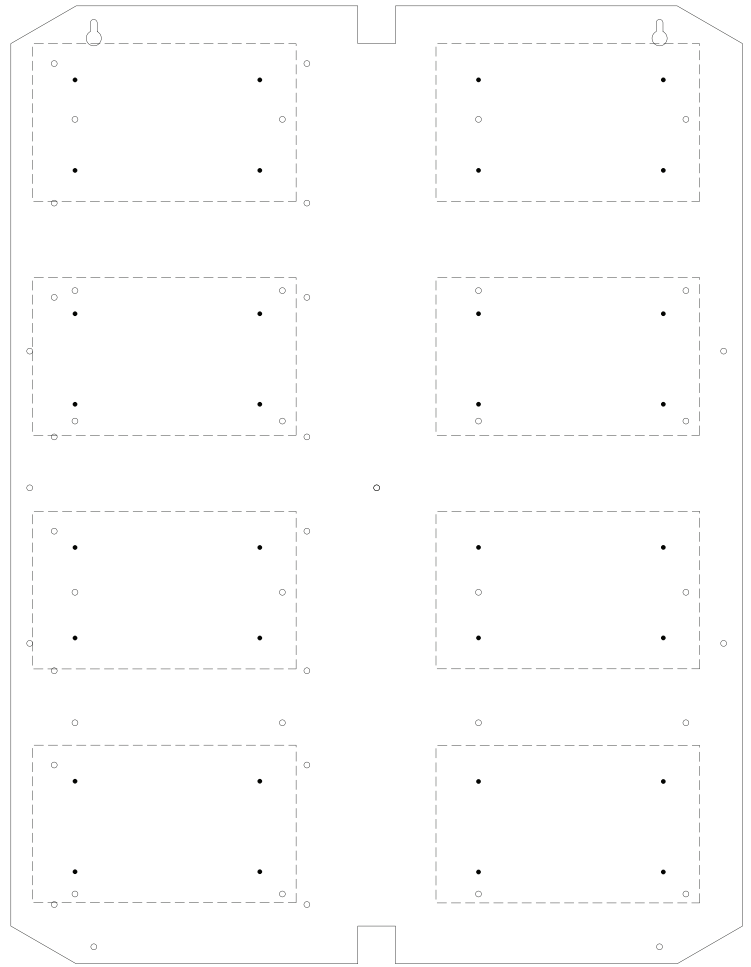
Fig. 3 - TV2 Altronix/HID/VertX Backplane
