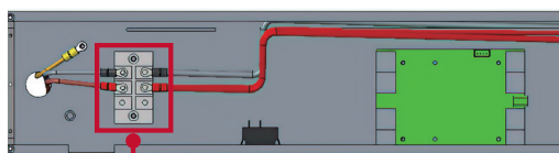
Deux(2) vis PWM 4x6mm
