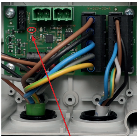
Figura 11: Scheda sensore
