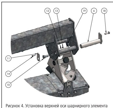
Рисунок 4. Установка верхней оси шарнирного элемента
