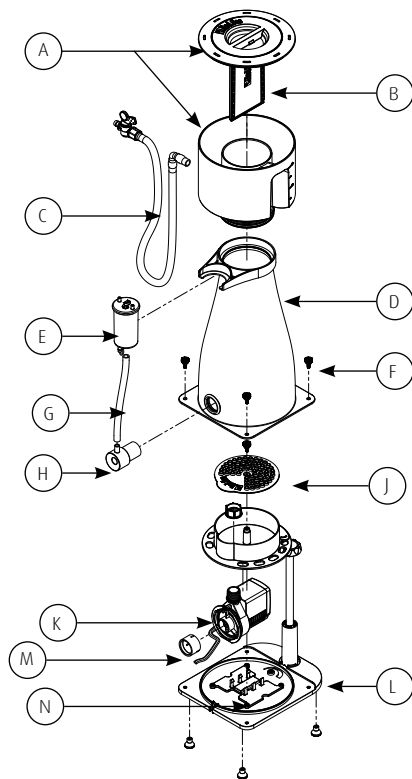
REEFER™ Skimmer 部品図
