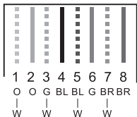
T568B
