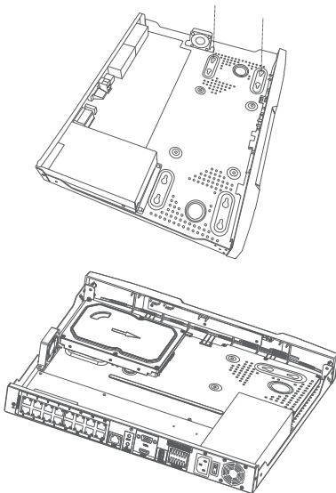
Gambar 6: Memasukkan Hard Drive
