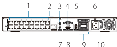
Figura 3: Connettori interfaccia pannello posteriore
