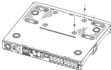
Figura 7: Fissaggio del disco rigido
