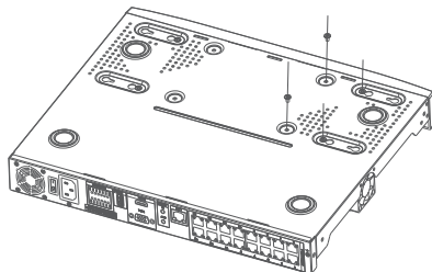
Figura 7: Fixando o Disco Rígido
