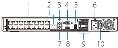
圖3：後面板連接介面
