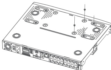
Figure 7 : Fixation du disque dur
