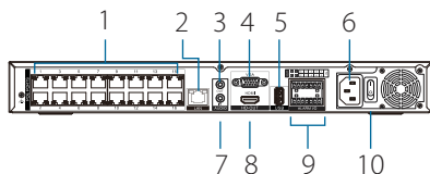
Figure 3 : Connecteurs d'interface de la face arrière
