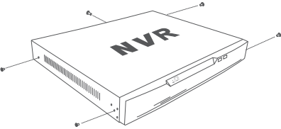
圖4：鬆開蓋子
