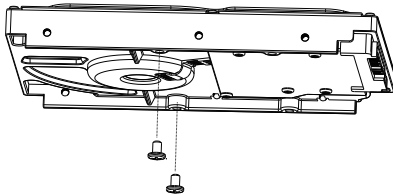
Figura 5: Fissaggio delle viti al disco rigido
