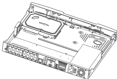
Малюнок 6: Встановлення жорсткого диска
