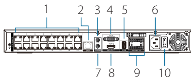
Малюнок 3: Інтерфейси задньої панелі
