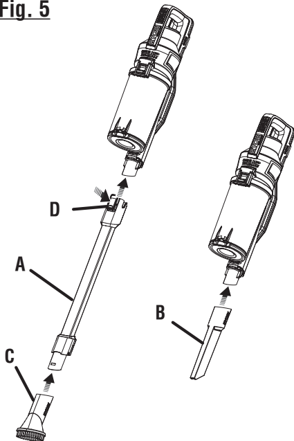
A - Extension wand (rallonge pour lance, tubo de extensión) B - Crevice tool (suceur plat, herramienta para hendiduras) C - Dust brush (brosse à poussière, cepillo para polvo) D - Locking tab (languette de verrouillage, orejeta de fijación)
