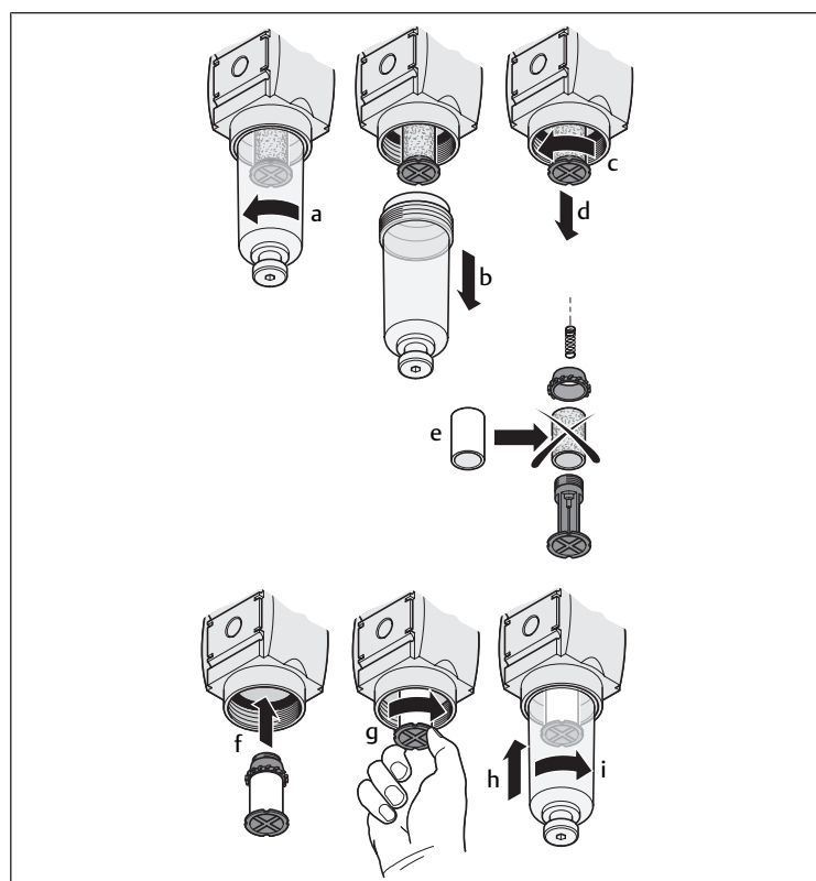
Fig. 5: Remplacement des filtres |
