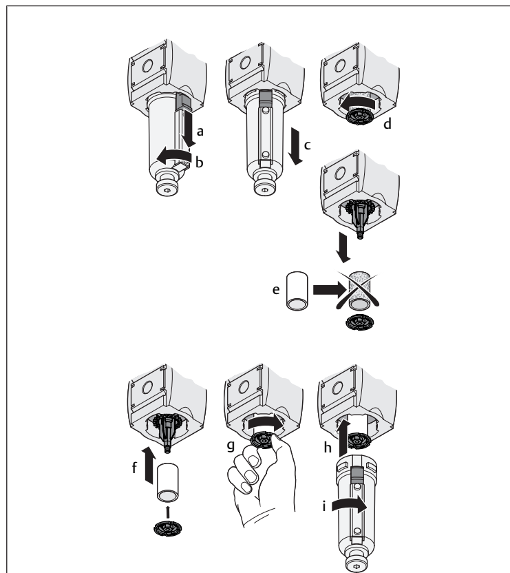
Abb. 6: Filter austauschen |
