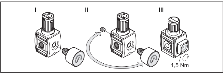
Abb. 1: I: Manometer montieren, II: Manometer austauschen | Serie AS2, AS3, AS5 III: Integriertes Manometer | Serie AS1
