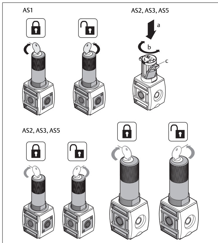
Abb. 3: Druckregelventil abschließen
