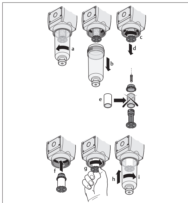
Abb. 5: Filter austauschen |
