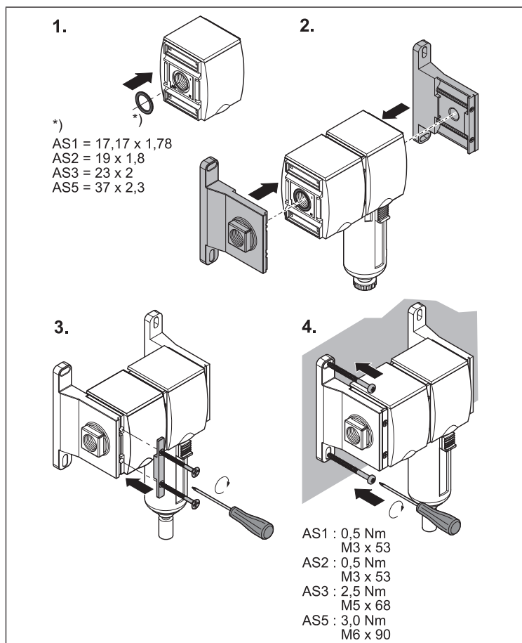
Bild 12: W05 | Blockmontering och fäste med blockmonteringssats
