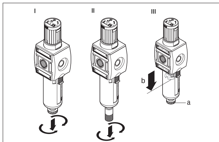
Fig. 4: Purge | Série AS1, AS2, AS3, AS5
