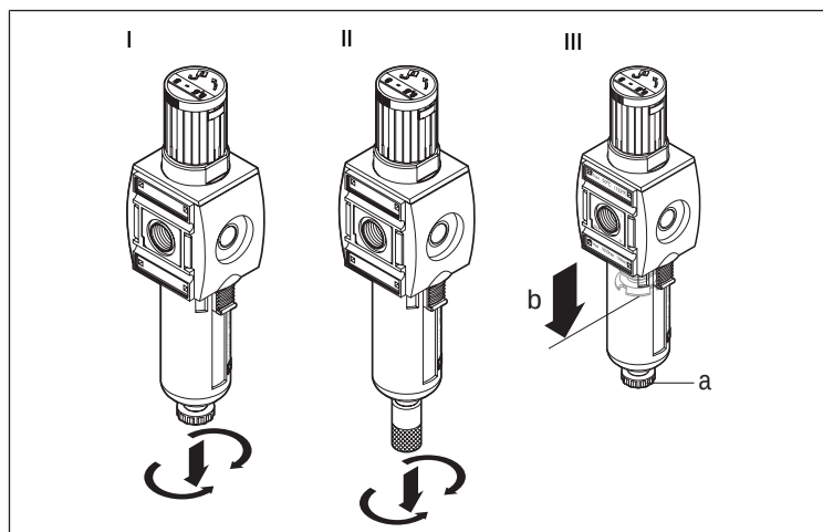
Fig. 4: Scarico di condensa | Serie AS1, AS2, AS3, AS5
