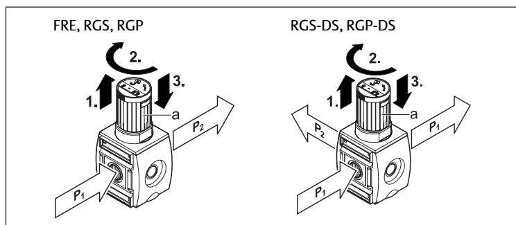
Fig. 2: Impostazione della pressione (P1 = pressione d'ingresso, P2 = pressione d'uscita) | Serie AS1, AS2, AS3, AS5
