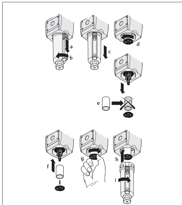
Bild 6: Byta filter |
