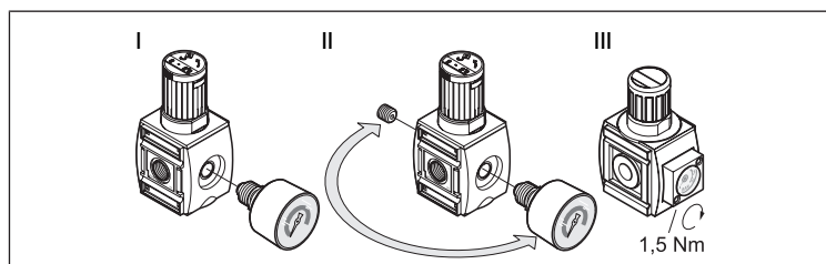
Fig. 1: I : monter le manomètre, II : remplacer le manomètre | Série AS2, AS3, AS5 III : manomètre intégré | Série AS1
