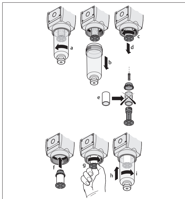
Bild 5: Byta filter |
