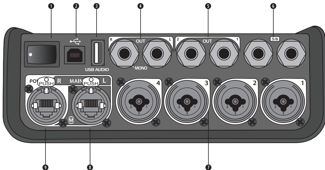
Abbildung 2. T4S Anschlussleiste
