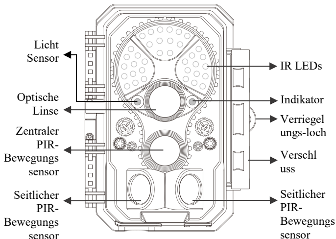
Abb. 1: Vorderansicht
