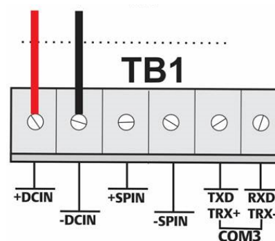
图8. 接线至直流电源
