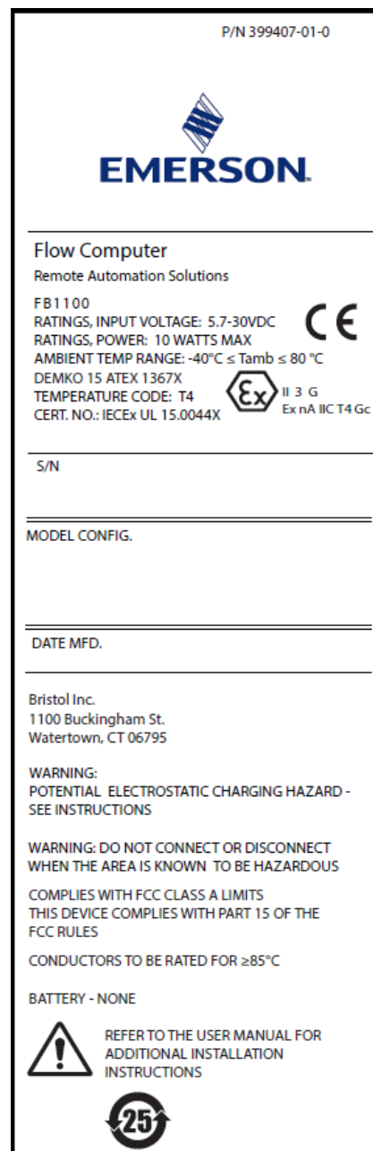
Figure 2. Étiquette Emerson FB1100 (anti-étincelles)
