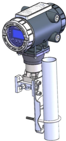
Figura 7. FB1100 su pala
