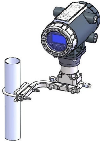
Abbildung 6. FB1100 mit Coplanar-Befestigung
