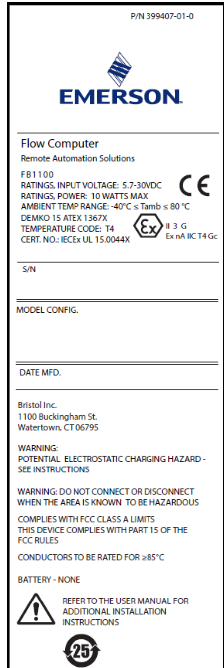
Figura 2. Etichetta FB1100 Emerson (a prova di scintille)
