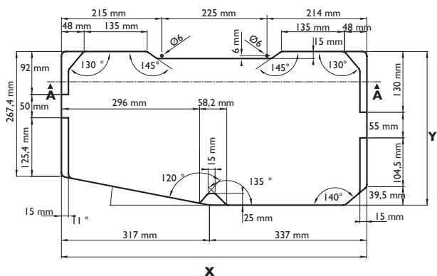
SEZA-A
