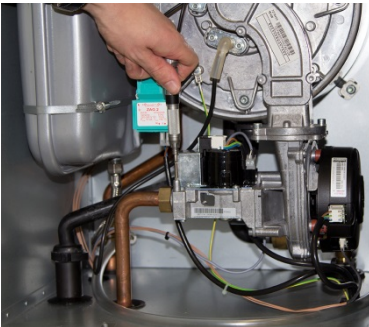
Abb. 4: Öffnen des Messstutzens
