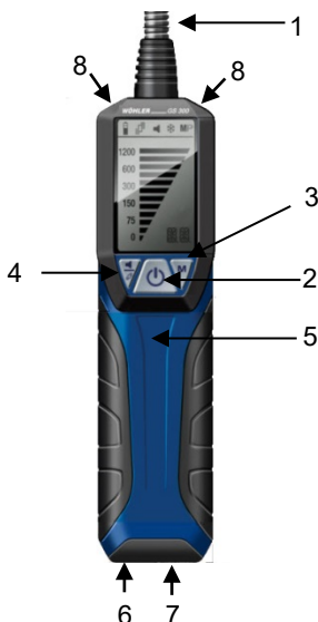
Afb. 23: Gasvoeler
