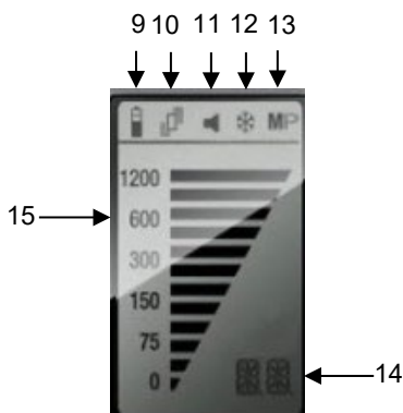
Afb. 24: Display gasvoeler
