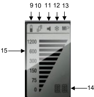
Afb. 24: Display gasvoeler
