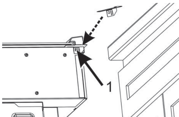
Figure 3 : Mise en place du cache-coin latéral droit
