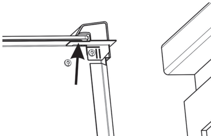
Figura 5: Cómo ajustar el tornillo
