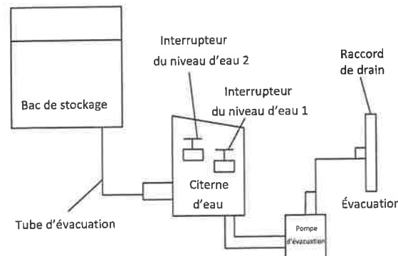
Diagramme schématique du système d'évacuation
