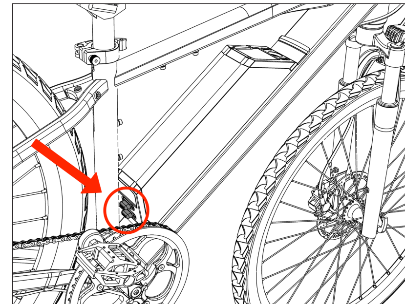
Fig. 8 - Fuse
