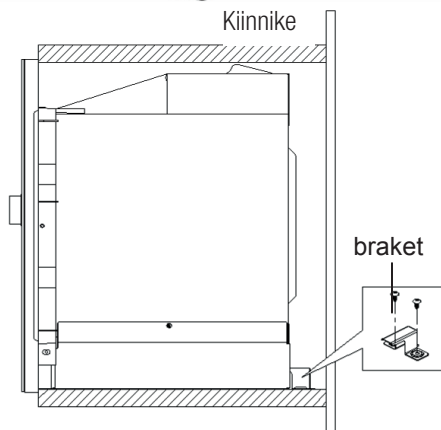
Kiinnike
