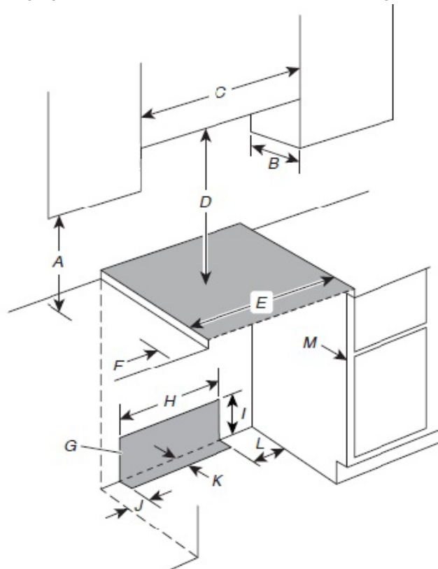
Découpe pour les commandes d'une cuisinière autoportante
