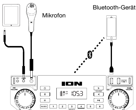
Vorderseite
