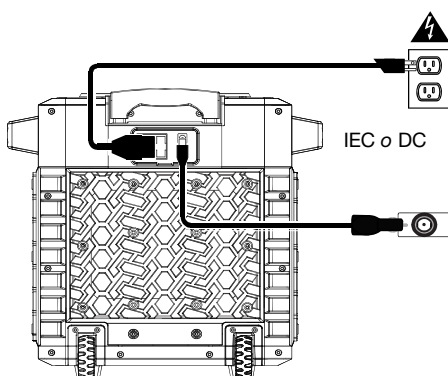
Pannello posteriore
