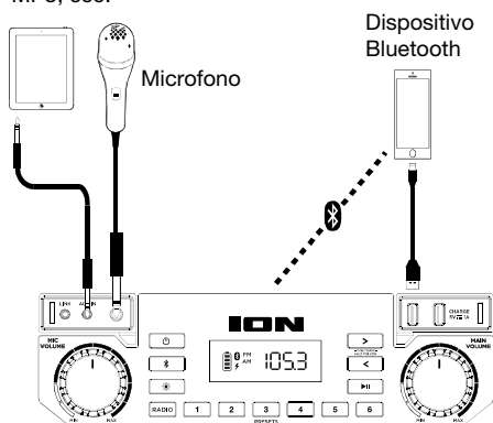
Pannello anteriore
