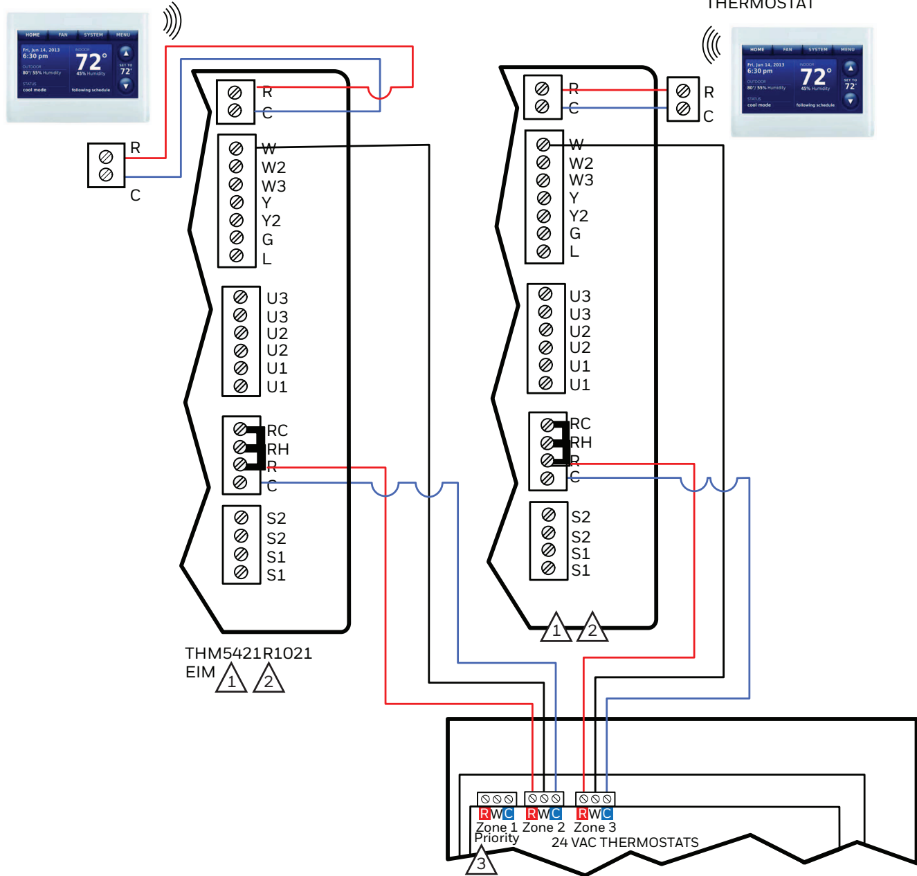
THX9421R5021 THERMOSTAT
