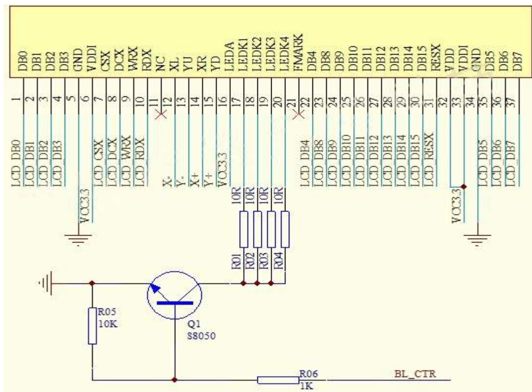
附图 6-1：显示屏 STP0240C1 MCU-8 位并口参考应用电路
