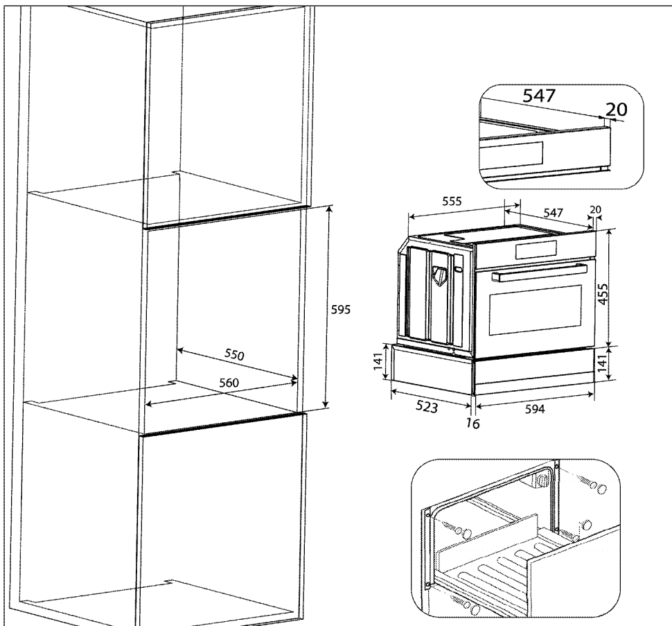
Verwarmingslade onder een compacte oven van 45 cm in een toreeneenheid
