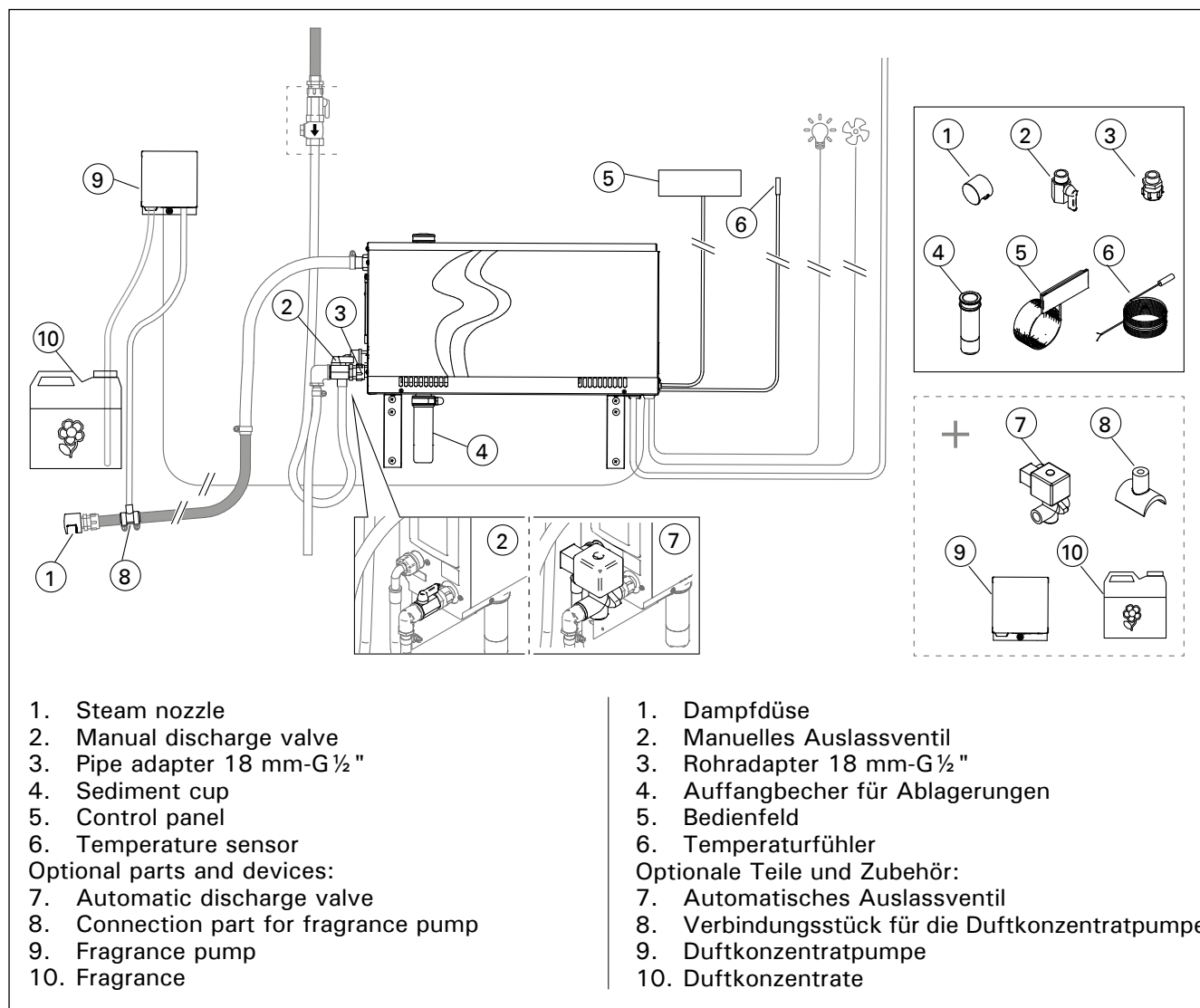
Figure 2. Steam generator system components Abbildung 2. Komponenten des Dampfgeneratorsystems
