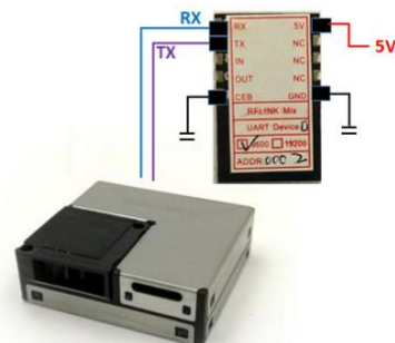
攀藤PM2.5模組
