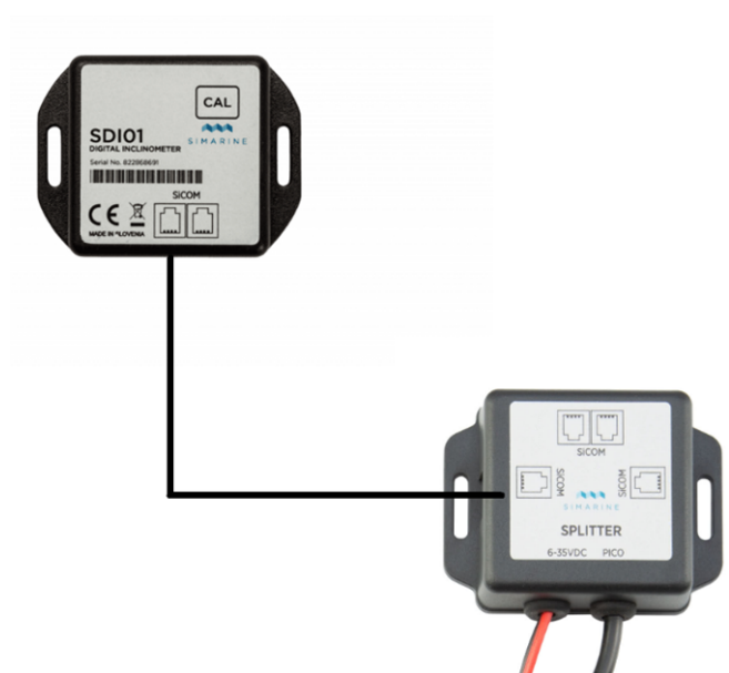
STANDARDVERKABELUNG - DIREKT ZUM SPLITTER
