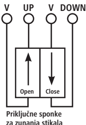
Priključne sponke za zunanja stikala
