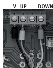
Ulkaisen näppäimen liittinkisko
