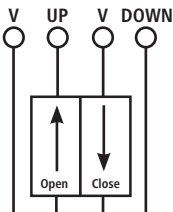
Zaciski przyłączeniowe do zewnętrznych przycisków
