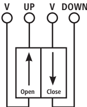
Přípojovací svorky pro externí vypínač
