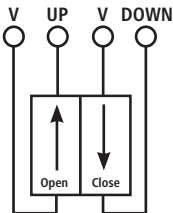
Bornes de raccordement pour bouton-poussoir externe
