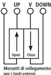
Morsetti di collegamento per i tasti esterni
