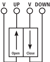
Terminais para interruptores externos
