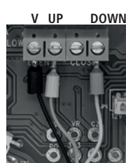
Přípojovací svorky pro externí vypínač
