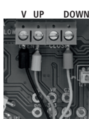
Priključne sponke za zunanja stikala
