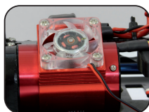
No. 130156 Refroidisseur moteur en Alu, actif avec ventilateur Cooling fins active with fan
