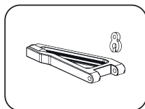
No. 505099 Directionnel avant haut Front upper suspension set
