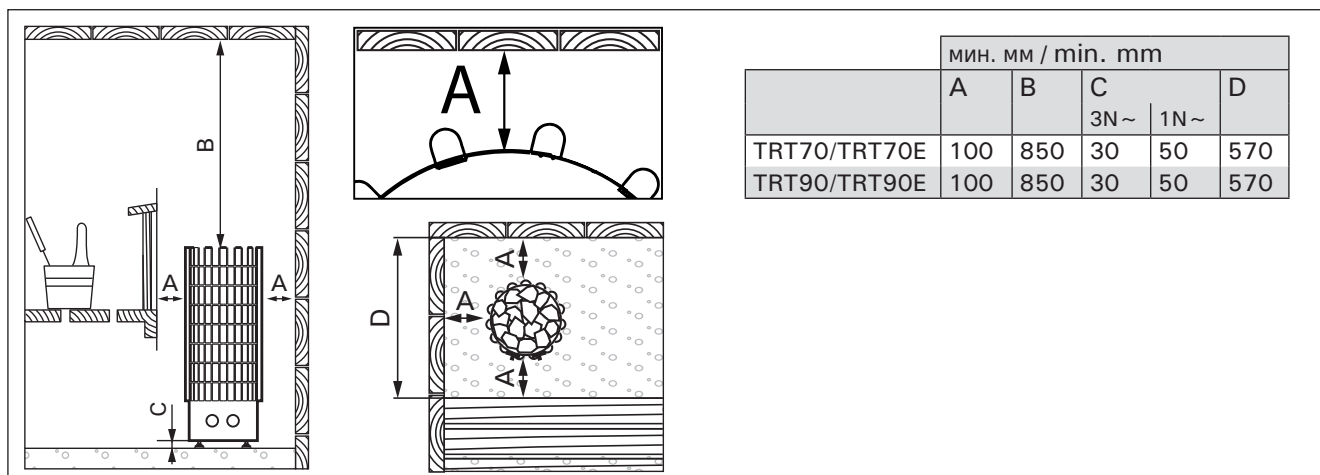
Рисунок 6. Расположение и безопасные расстояния (все размеры приведены в миллиметрах) Joonis 6. Ohutuskaugused (kõik mõõtmekillimeetrites)
