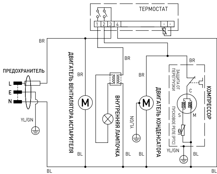
Электрическая схема (233900)
