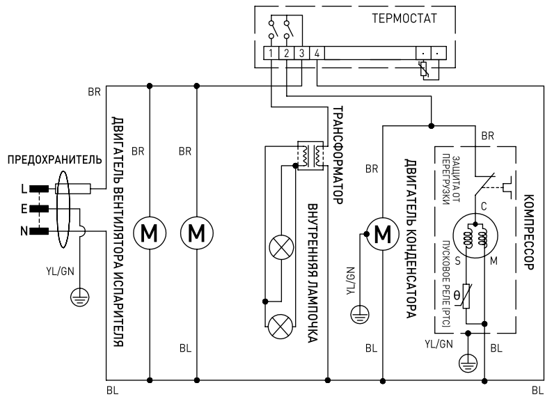
Электрическая схема [235829]
