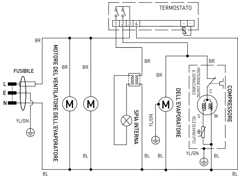
Schema elettrico [233917]
