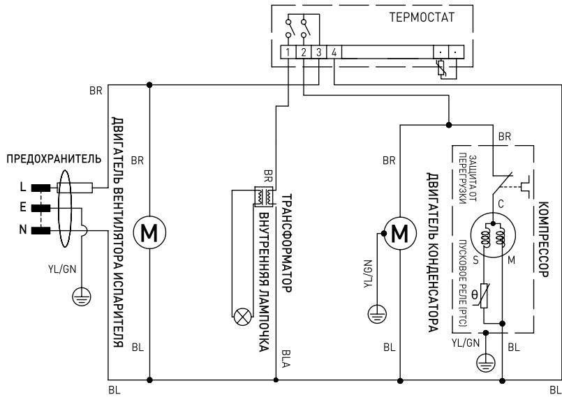
Электрическая схема (233900)
