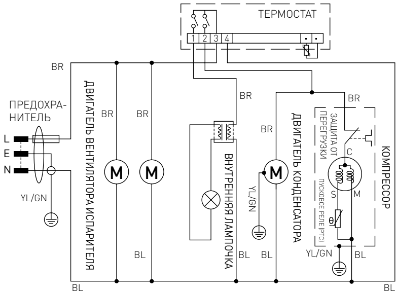
Электрическая схема [235829]
