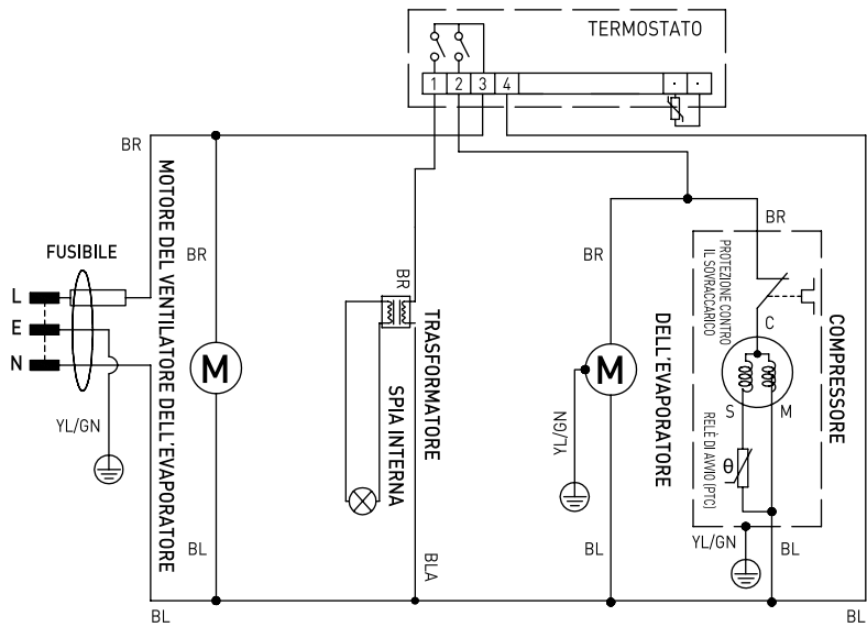
Schema elettrico [233917]
