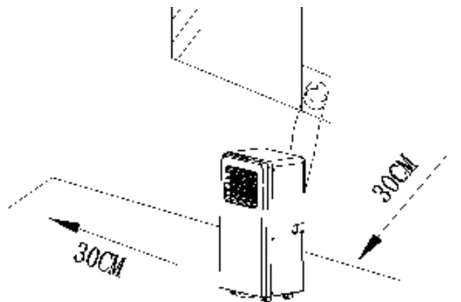
A kivezetőcső felszerelése
