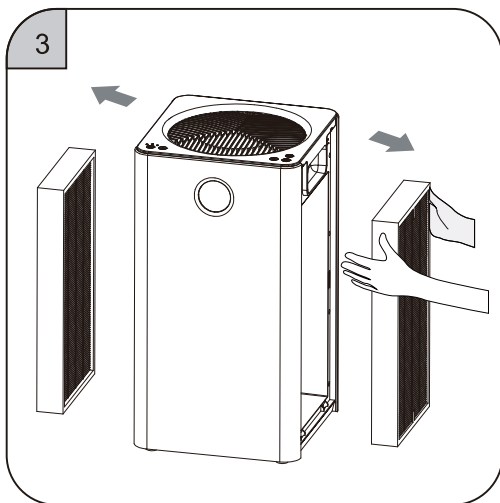
③ Estrarre il nuovo schermo filtrante con pellicola di plastica nella macchina.
