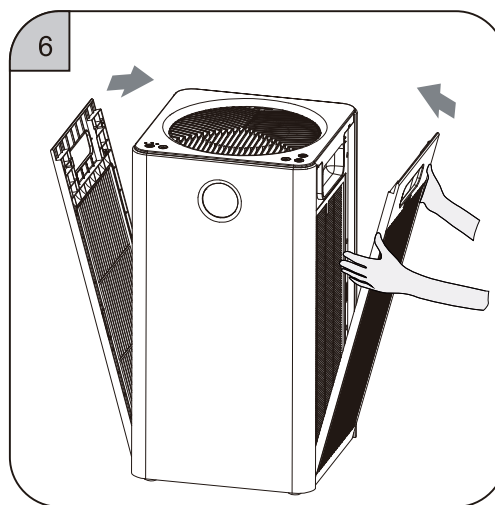
⑥ Installare il coperchio del filtro.
