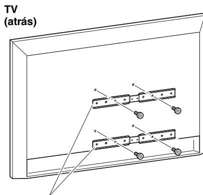
Suporte de montagem do monitor (horizontal)
