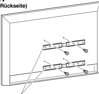
(Waagerechte) Bildschirmhalterung
