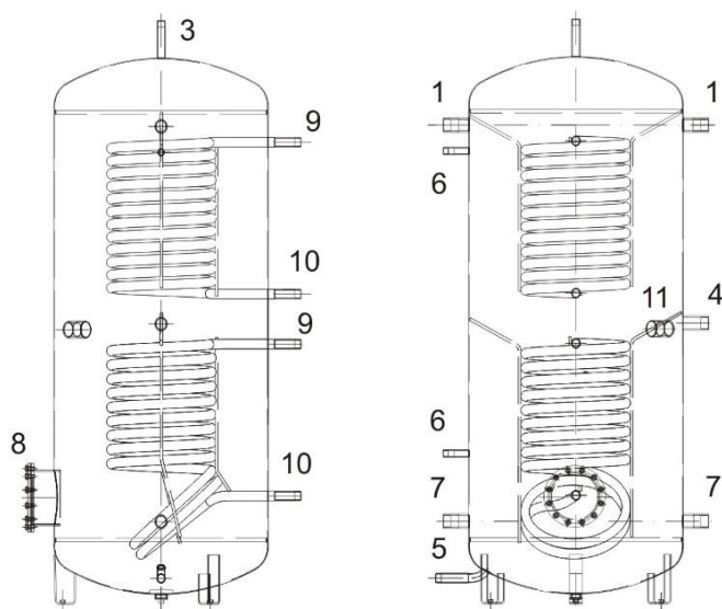
NAD v4 - csak alsó hőcserélő NAD v5 - két hőcserélő
