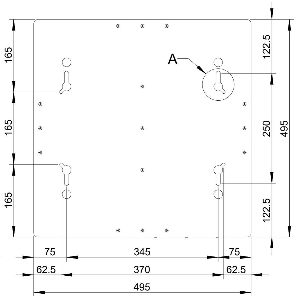
Rückansicht/ Rear view
