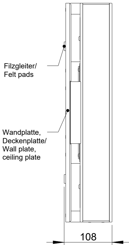
Seitenansicht/ Side view
