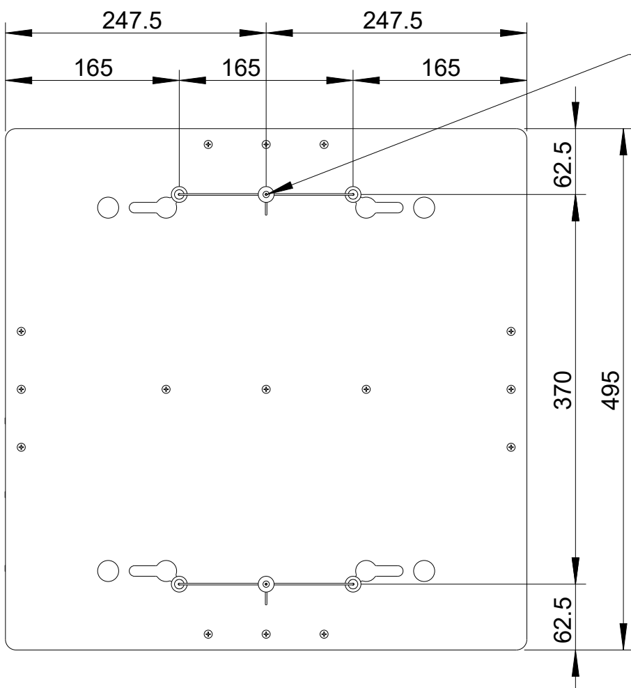
Draufsicht/ Top view
