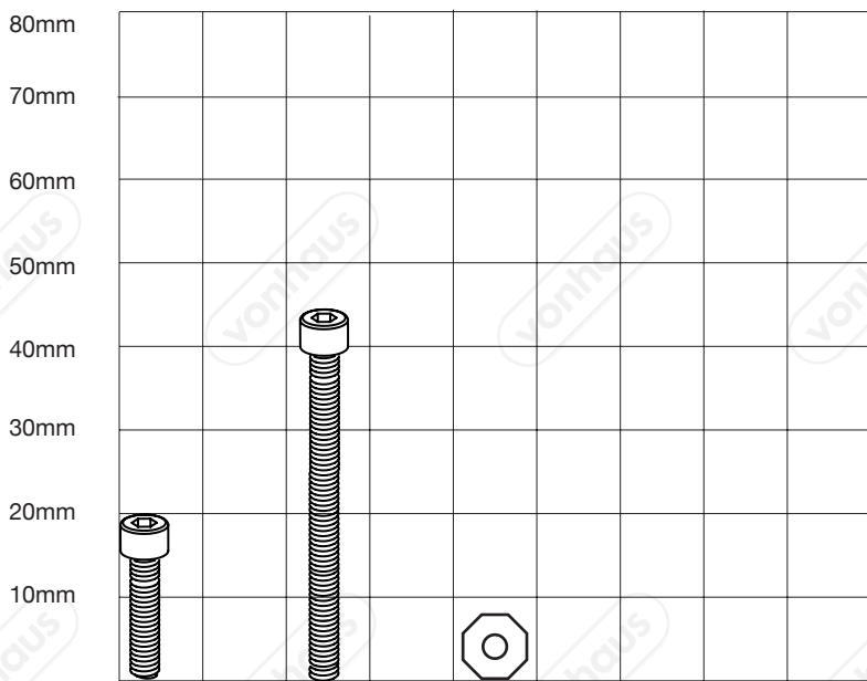
A: M5 x 20mm (x4) B: M5 x 44mm (x1) C: 8mm (x5)
