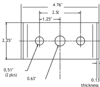
DSXF1 DSXF2 YOKE
