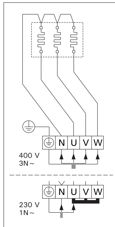
Рисунок 9. Подключение каменок PI-E Joonis 9. Kerise PI-E elektriühendused
