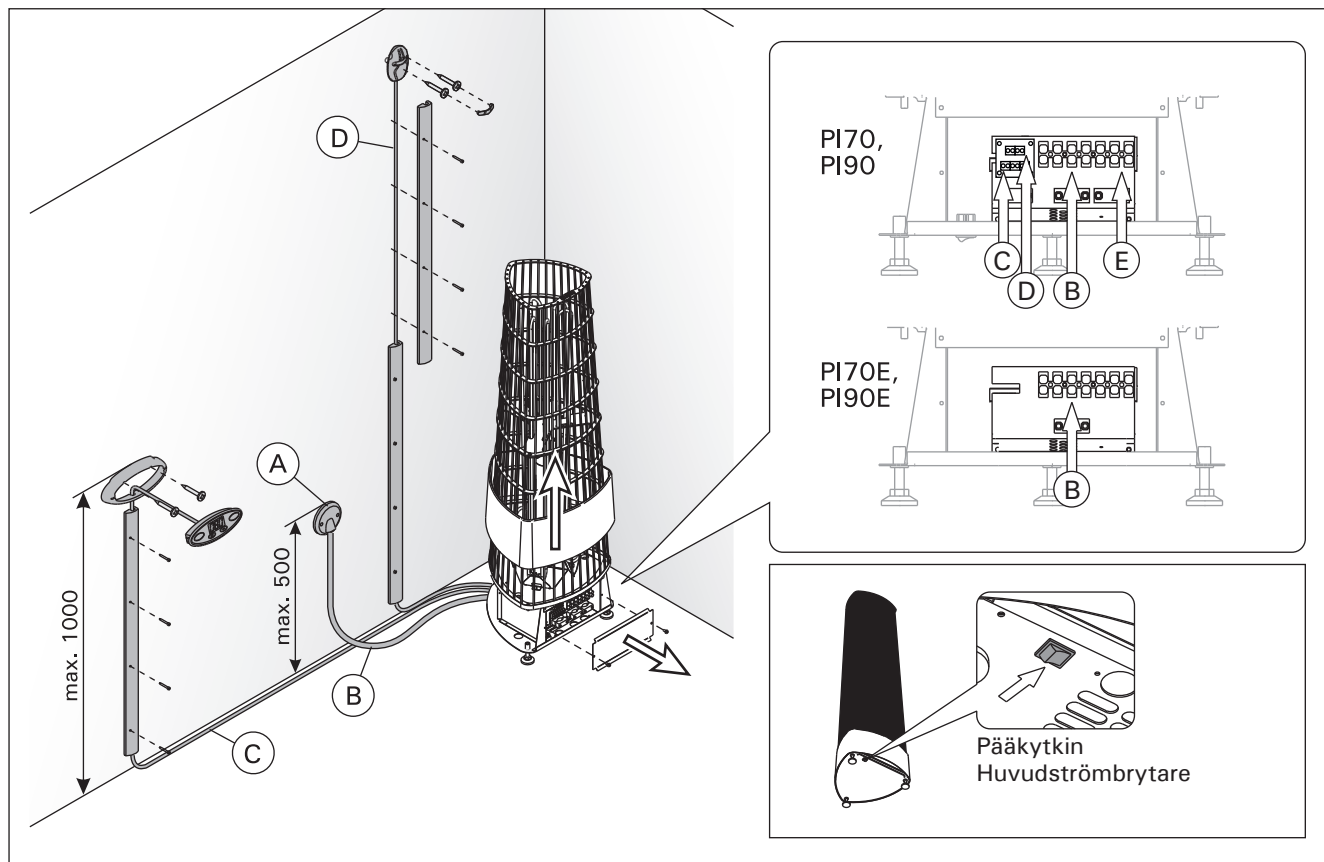
Kuva 7. Sähkökytkennät (mitat millimetreinä) Bild 7. Elinstallation (mått i millimeter)
