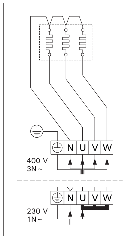
Kuva 9. PI-E-kiukaan sähkökytkennät Bild 9. Elinstallationer av PI-E-aggregat
