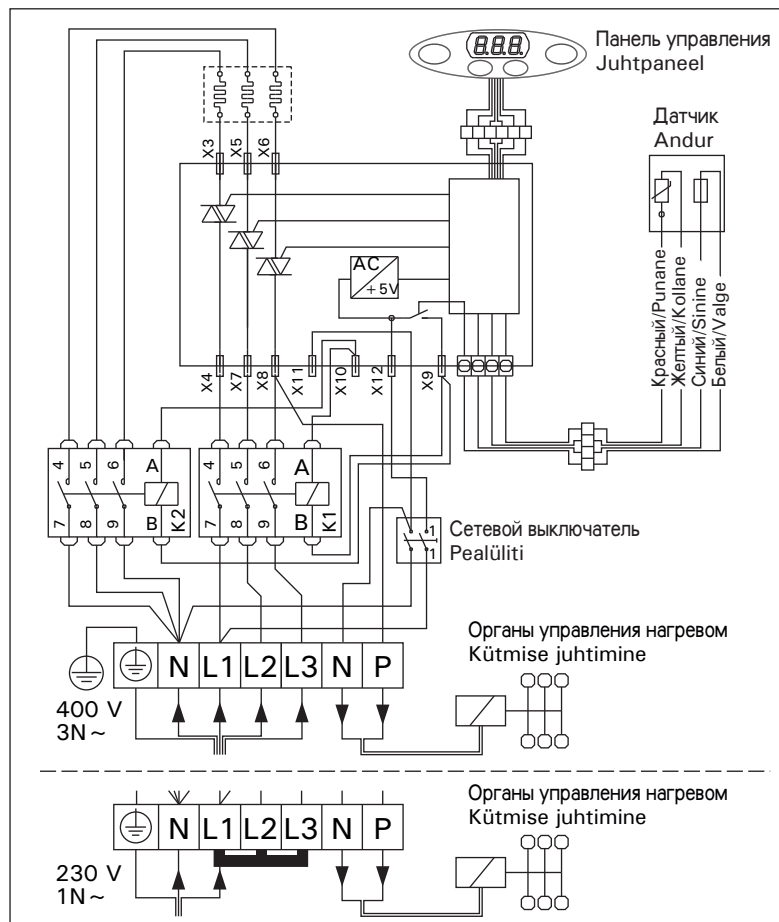
Рисунок 8. Подключение каменок PI Joonis 8. Kerise PI elektriihendused
