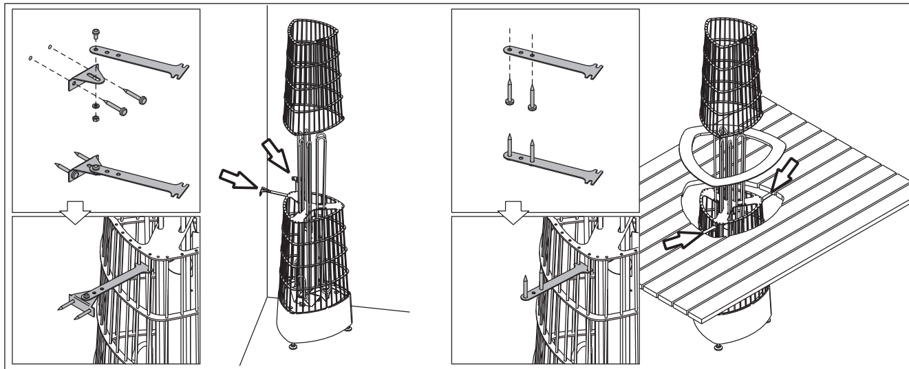
Kuva 11. Kiukaan kiinnittäminen kiinnityssarjojen avulla
