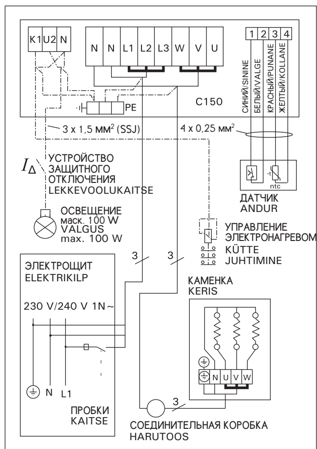
Рисунок 10b. Электромонтаж пульта управления C150 и каменки PI-E (подключение в 1-фазной сети)
