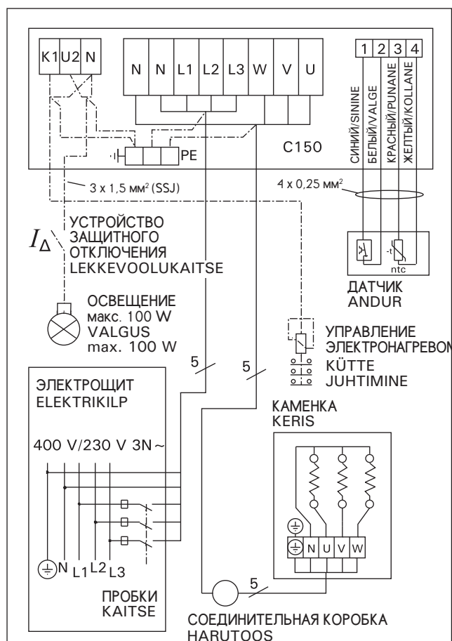
Рисунок 10а. Электромонтаж пульта управления С150 и каменки PI-E (подключение в 3-фазной сети)
